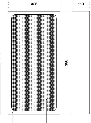
Opnameframe Filtermatte
